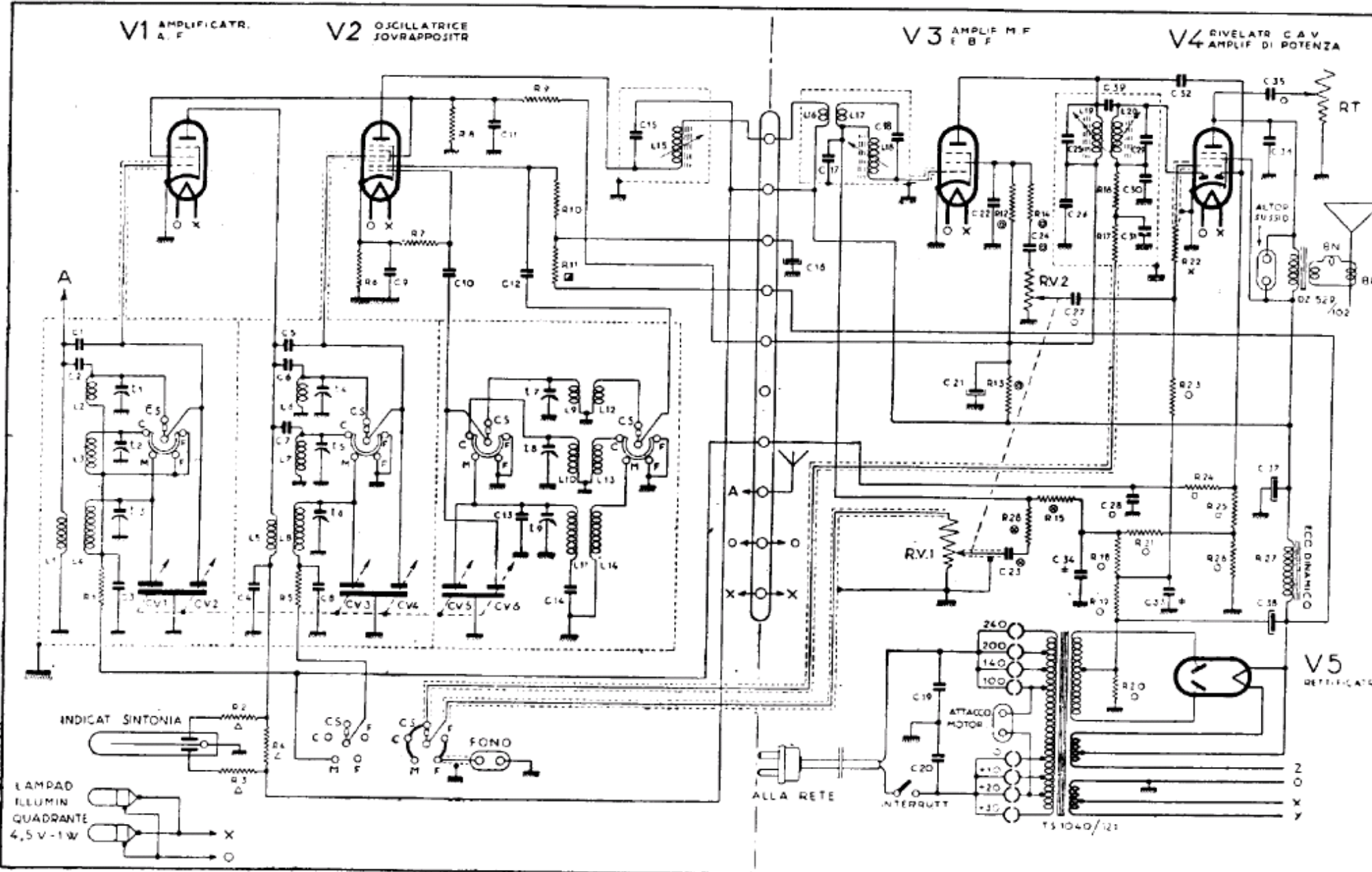
137. — PHONOLA (S. A. FIMI). — Mod. 515 e 516. — 11-21,7 kHz, 5,7-11,4 kHz, 500-1500 kHz. — Produzione 1937-1938. — Media frequenza: 470 kHz.
